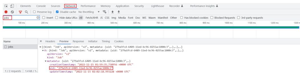
图 7-1 获取 job_id
